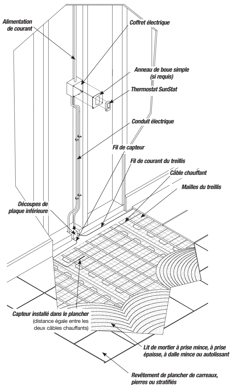
Disposition générale de l'installation du treillis SunTouch
