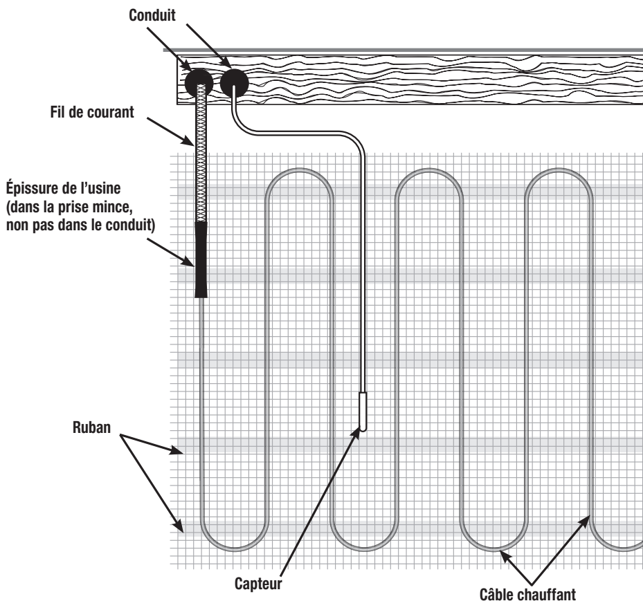
Vue de haut en bas du treillis et le capteur entrant dans le mur.
