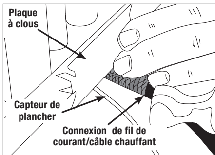
Placez une plaque à clous métallique sur le point de transition pour protéger le fil de courant et le fil du capteur.
